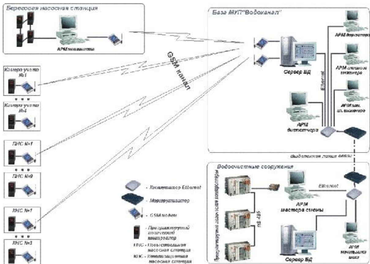
Пример структурной схемы диспетчеризации объектов водоснабжения и водоотведения
